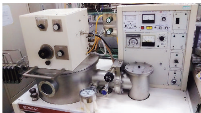
図3 本研究で用いたスパッタ装置
