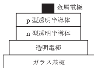
図1 透明太陽電池の構造
