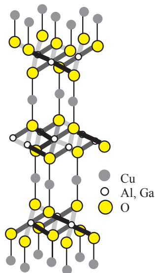
図2 デラフォサイト結晶
